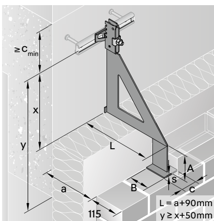
Einzelkonsole JVAeco+ NA mit tiefgesetztem Konsolaufleger
