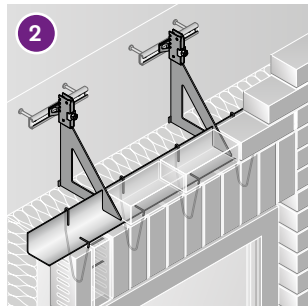
Öffnungen: Verblenderkonsole JVAeco+ F/FAR (s. S. 18–19)
