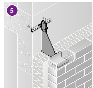
Dehnungsfuge und Randbereich: Verblenderkonsole JVAeco+ E/EA (s. S. 17)
