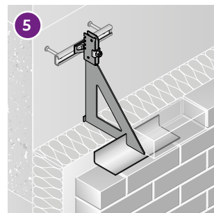
Dehnungsfuge und Randbereich: Verblenderkonsole JVAeco+ P/PAR (s. S. 16)
