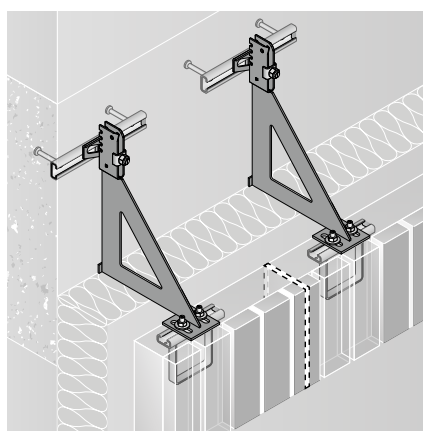
Abhängesystem JFT+ für die Abhängung von Fertigteilstürzen
