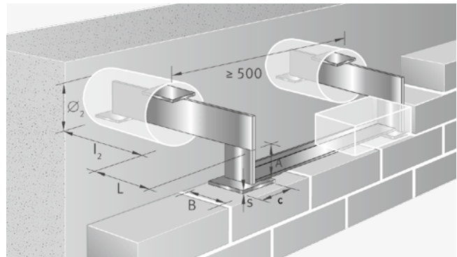
Einmörtelkonsole JMK+ NA
