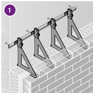
Normalwandbereich: Verblenderkonsolen JVAeco+ N/NA (s. S. 12–13) u. JVAeco+ P/PAR (s. S. 16)
