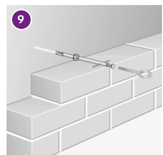
Gerüstssicherung: Gerüstanker JGA+ (s. S. 40–41)
