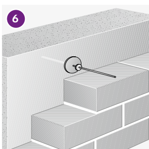
Sicherung des Verblendmauerwerks gegen Knicken: Luftschichtanker JLA (s. S. 34–35)
