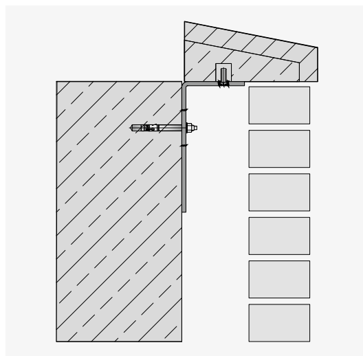
Sonderkonsole FB-SX mit gezahntem Langloch und einer horizontalen Lagesicherung
