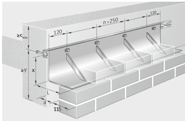
Winkelkonsole L-DF+ mit Diagonalaussteifung
