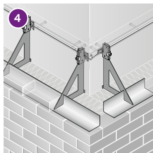
Außenecke ohne Dehnungsfuge: Verblenderkonsole JVAeco+ F (s. S. 18)
