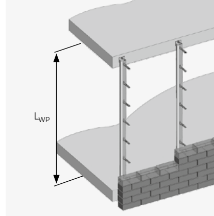
Windpost JWP und Maueranschlussanker JMA
