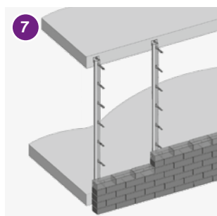
Horizontale Lagesicherung: Windpost JWP (siehe Seite 37) und Maueranschlussanker JMA (s. S. 38)
