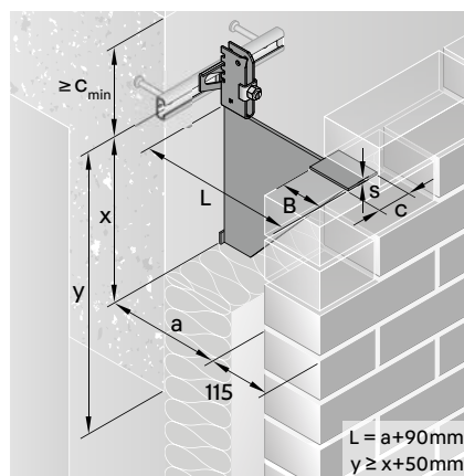
Einzelkonsole JVAeco+ NU mit hochgesetztem Konsolaufleger
