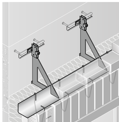
Unsichtbare Abfangung über Fensteröffnung mit JVAeco+ F, Rollschichthaltern JRH und Edelstahldraht ESD
