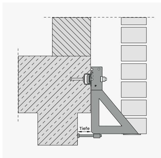
Sonderkonsole mit Druckschraube zur Tiefenjustierung
