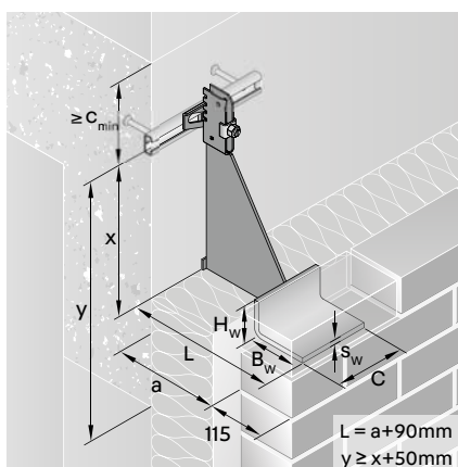
Einzelkonsole JVAeco+ E
