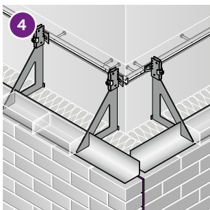
Außenecke mit Dehnungsfuge: Verblenderkonsole JVAeco+ F (s. S. 18)
