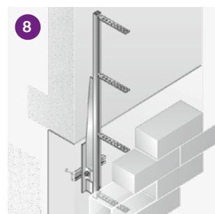
Abfangungen im Attikabereich: Attika-Verblendanker JAV (siehe Seite 36) und Maueranschlussanker JMA (s. S. 38)
