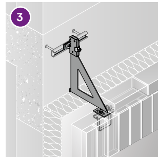
Öffnungen mit Fertigteilstürzen: Verblenderkonsole JVAeco+ NFT/NAFT (s. S. 24)
