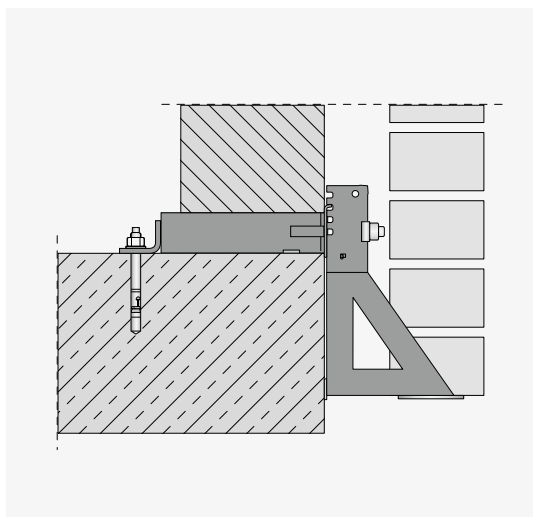
Standardkonsole JVAeco+ mit Zusatzbauteil Typ JVAeco+ ZB zur Montage auf dünnen Decken
