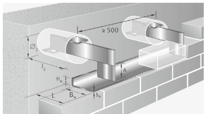
Einmörtelkonsole JMK+ FAR
