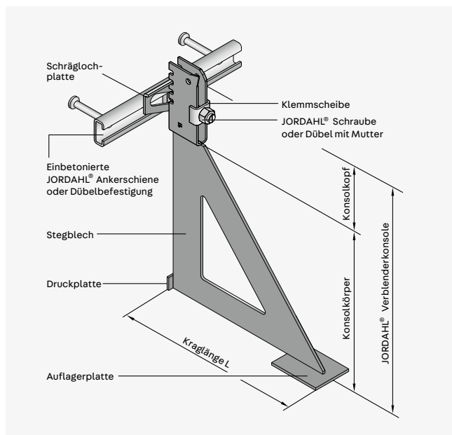
Die JORDAHL® Verblenderkonsole JVAeco+ besteht wie alle JORDAHL® Systeme für Verblendmauerwerk komplett aus Edelstahl.
