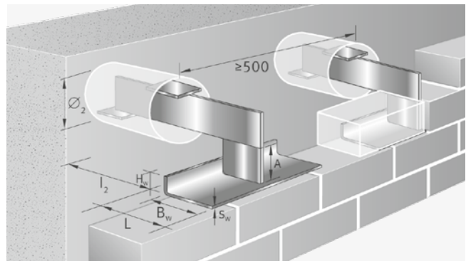
Einmörtelkonsole JMK+ PAR
