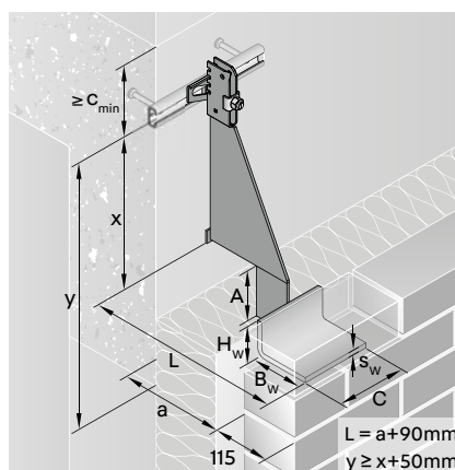
Einzelkonsole JVAeco+ EA mit tiefgesetztem Konsolaufleger
