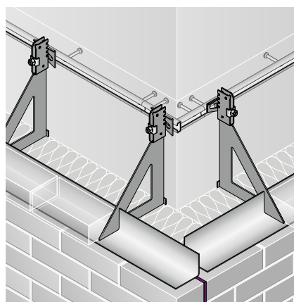
Ausführung einer Außenecke mit vertikaler Dehnungsfuge mit JORDAHL® Verblenderkonsolen JVAeco+ F
