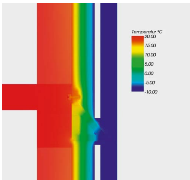
Temperaturverlauf mit JORDAHL® Verblenderkonsole JVAeco+ und JORDAHL® Thermomanschette JTM
